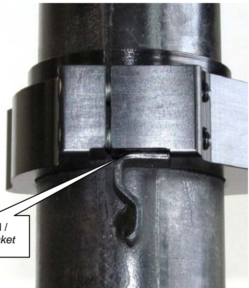
Dichtung der Gewindehülse einfetten. Seal the threaded sleeve grease.
